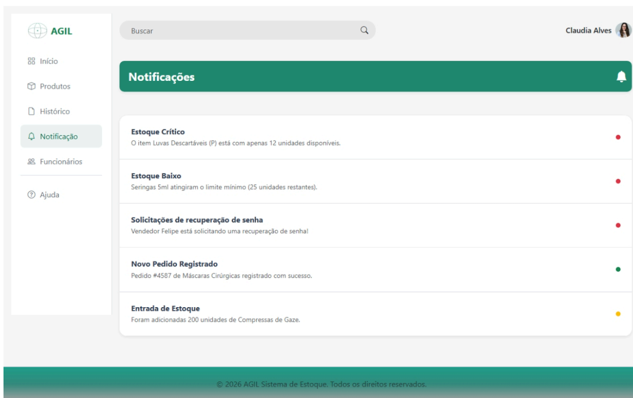
Figura 15 - Tela Notificações
