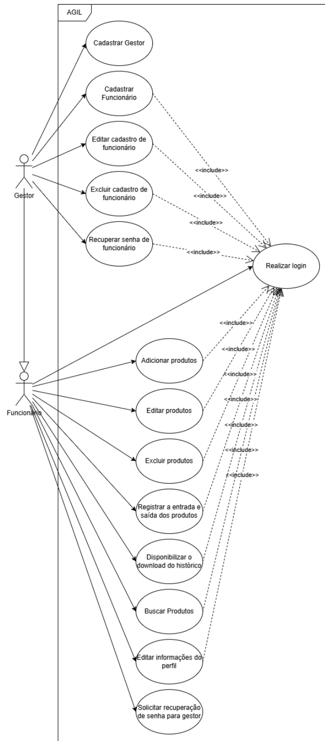
Figura 1 – Diagrama de Casos de Uso.
