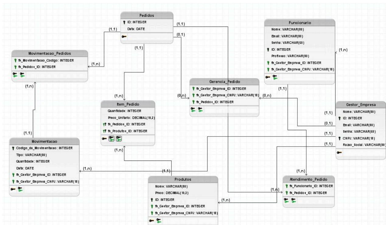
Figura 3 - Modelo Lógico
