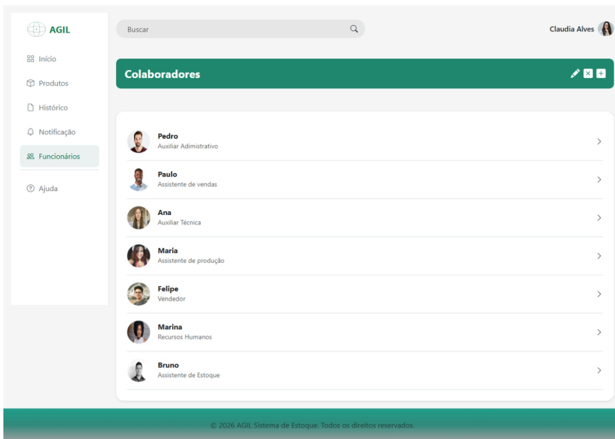
Figura 16 - Tela Funcionários
