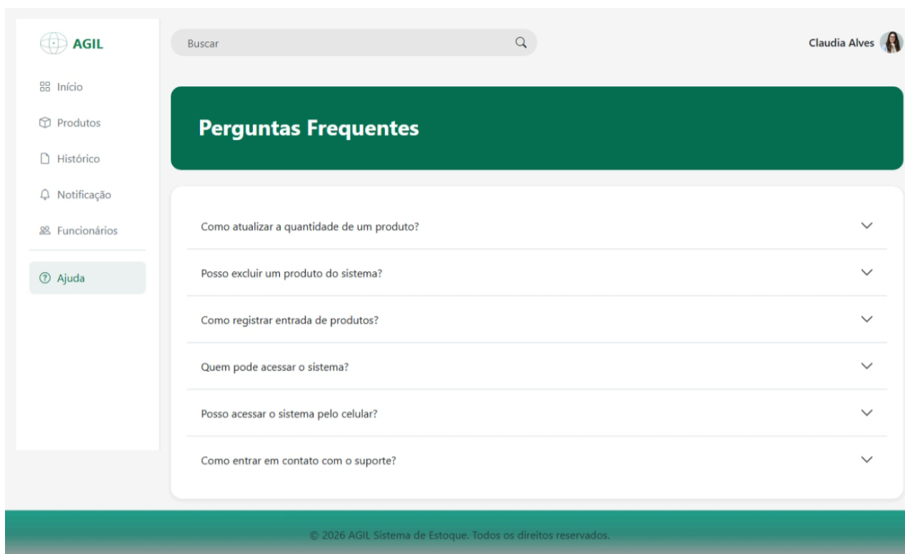
Figura 17 - Tela Ajuda
