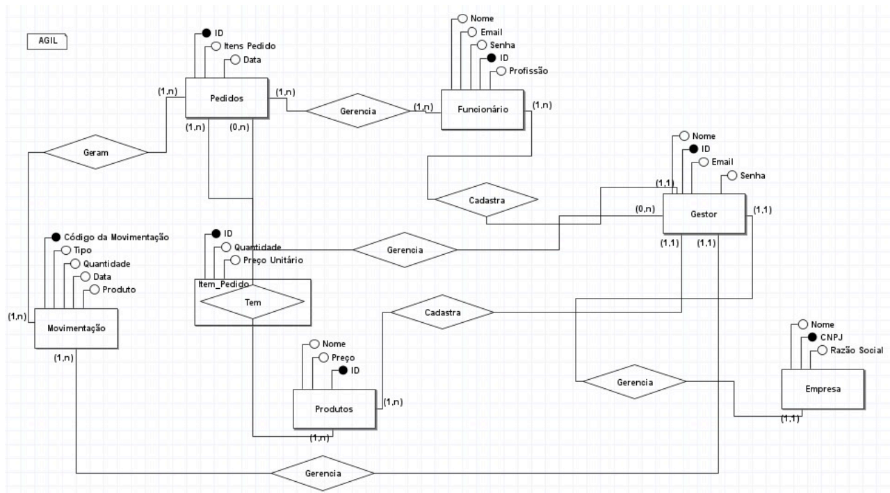
Figura 2 - Modelo Conceitual
